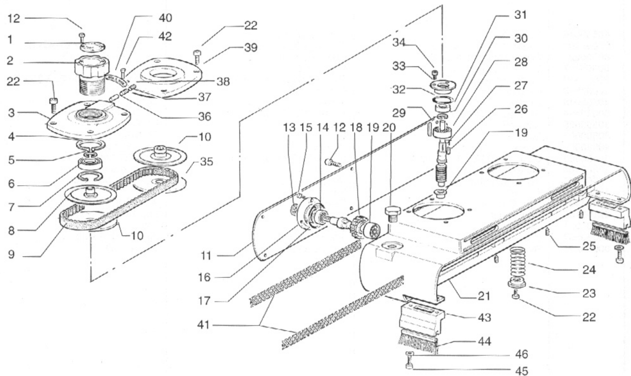
ABB. 1 - GEHÄUSE-EINHEIT TAB. 1 - BATY GROUP PL. 1 - ENSEMBLE BATY
