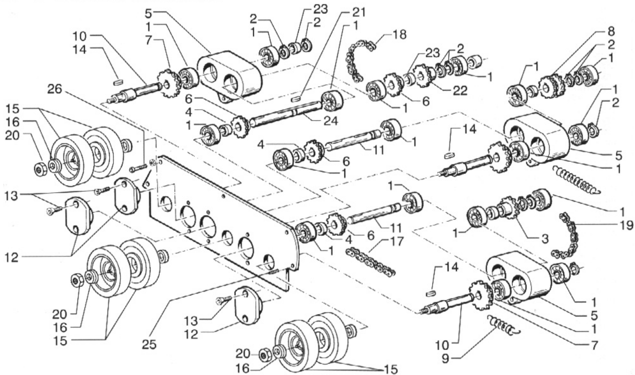
ABB. 2 - ÜBERTRAGUNGSEINHEIT TAB. 2 - TRANSMISSION GROUP PL. 2 - ENSEMBLE TRANSMISSION
